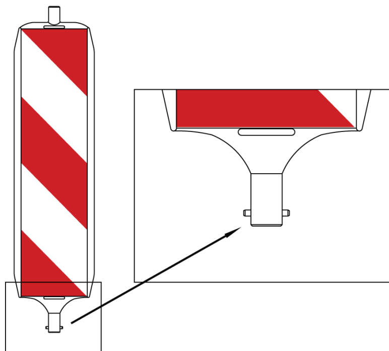
Пример могуће монтаже вертикалне запреке - монтажни систем „окрени и закључај“
