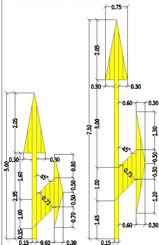
Стрелица за смер право и десно
