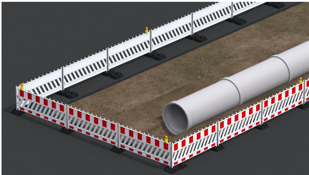
Слика 91. Ограђивање зоне радова хоризонталним запрекама VII-2.4 за дубине ископа преко 1,25 m
