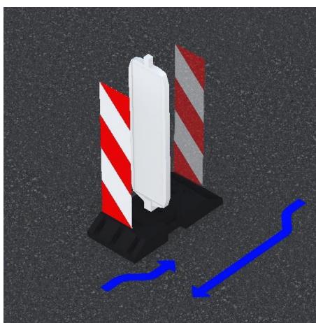
Слика 11. VII-3.1/VII-3.2 (ДДЛ) Двострана десна/лева вертикална запрека
