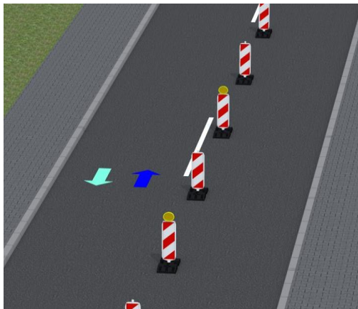
Слика 18. Затварање једне коловозне траке
