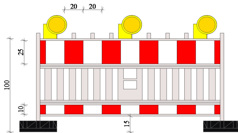
Хоризонтална запрека VII-2.2 (двострука)
