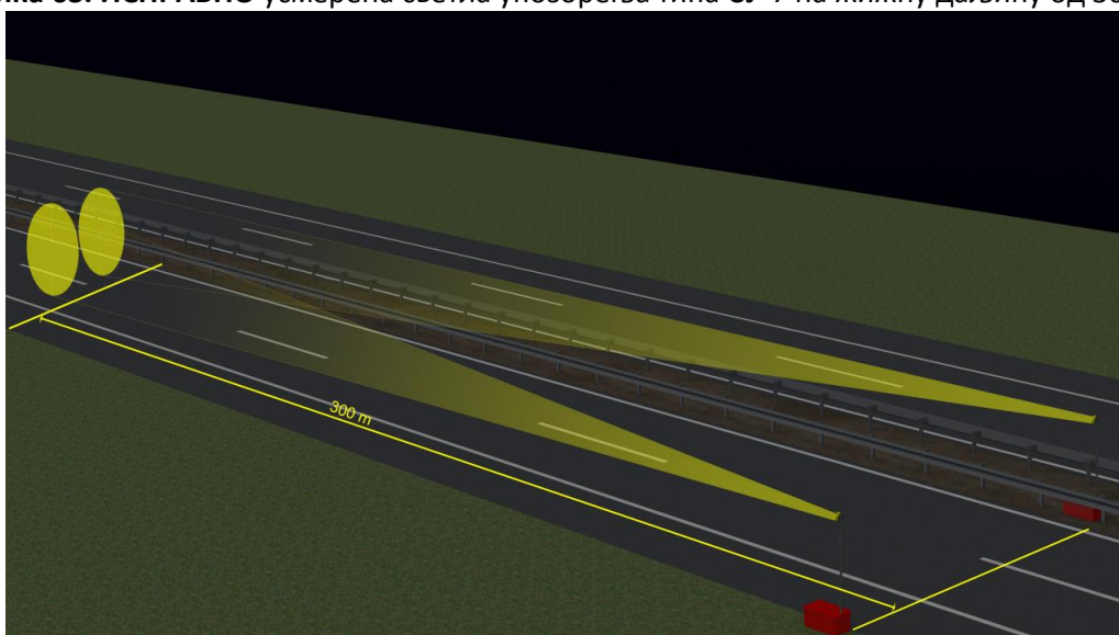
Слика 64. ИСПРАВНО усмерена светала упозорења типа СУ-7 на жијну даљину од 300 m
