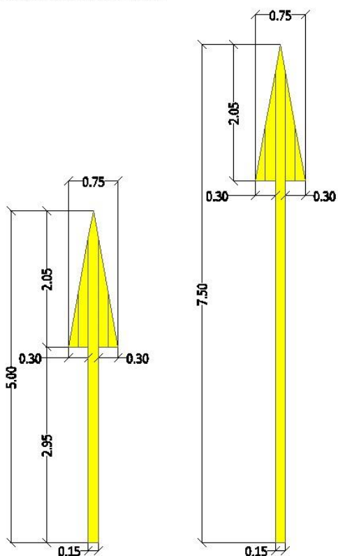
Стрелица за смер право
