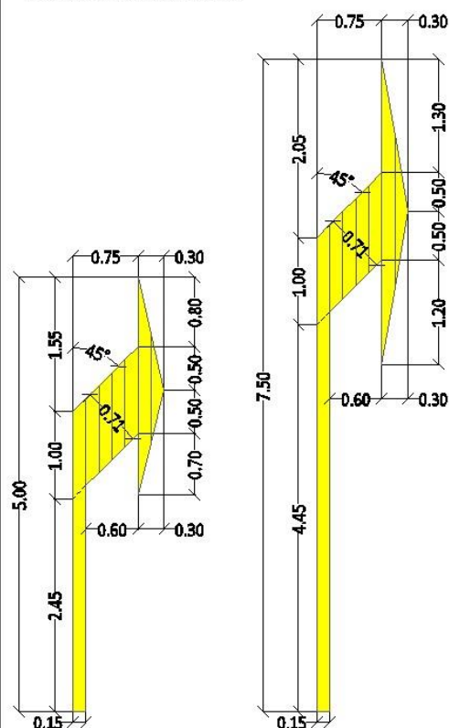
Стрелица за смер десно
