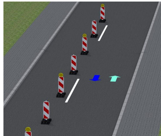
Слика 19. Поглед из супротног смера
