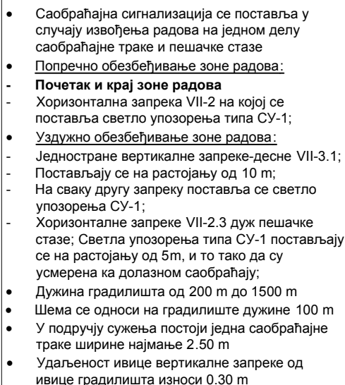
Одвијање једносмерног саобраћаја на суженом коловозу са смањењем броја трака
