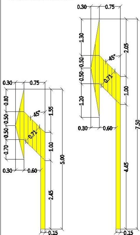
Стрелица за смер лево
