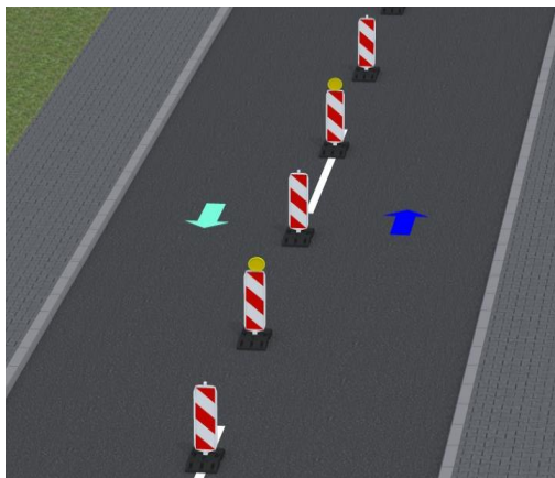
Слика 20. Поглед из једног смера
