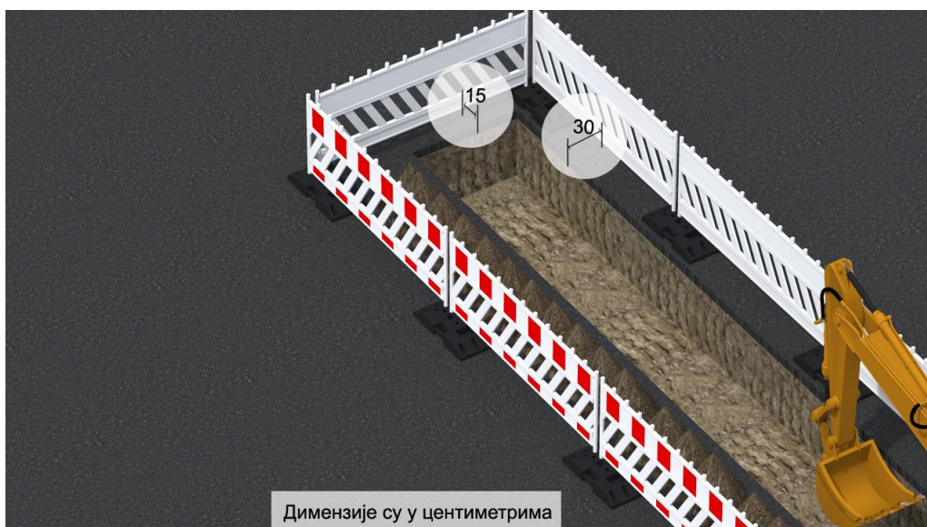
Слика 92. Минимална удаљења средстава за ограђивање од ивица ископа дата у cm
