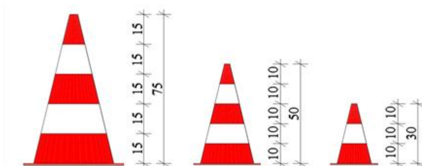
Основне димензије саобраћајних чуњева висине 30 cm, 50 cm и 75 cm
